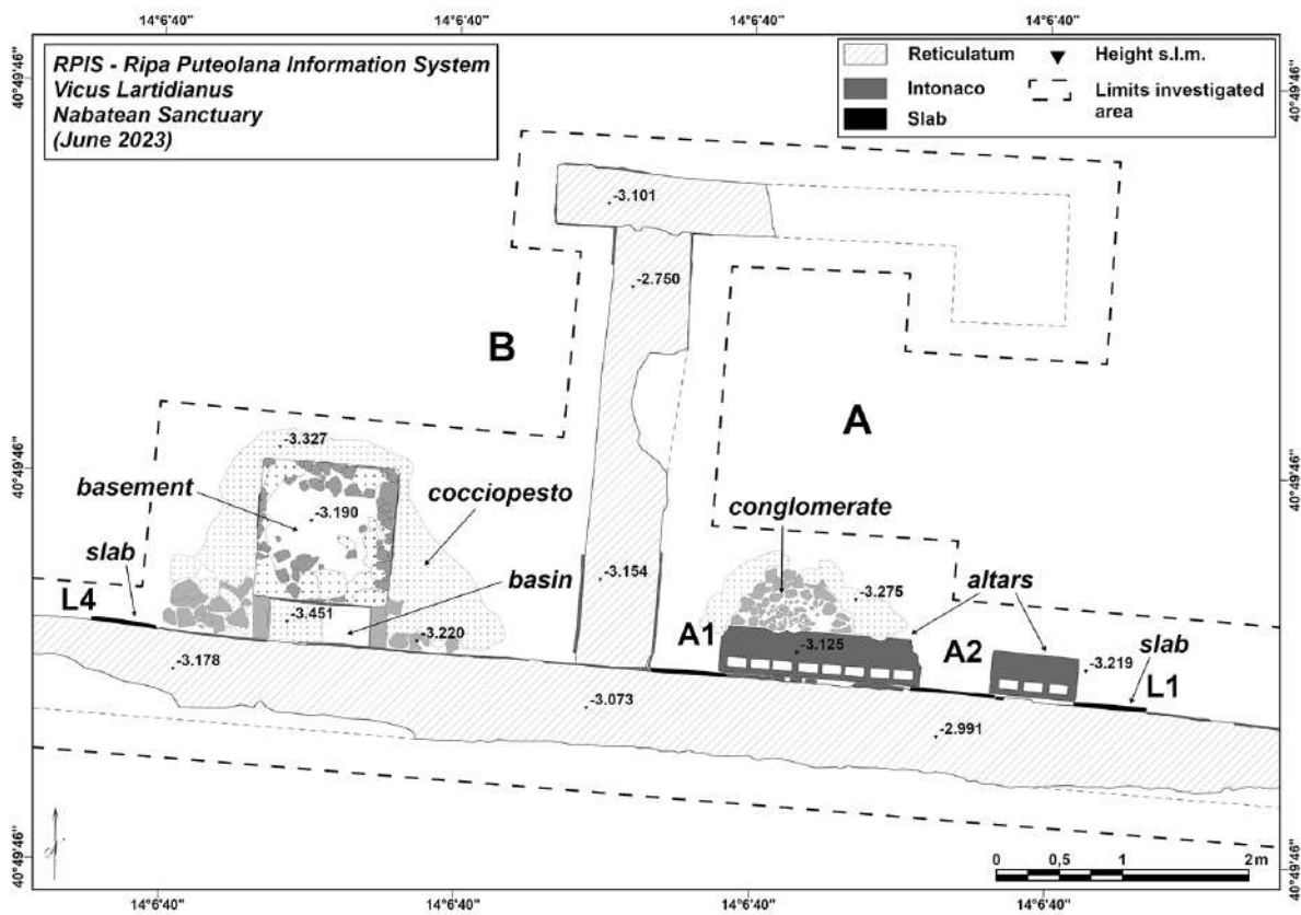
Puteoli. Planimetria dell'area investigata nel tempio sommerso dei Nabatei
